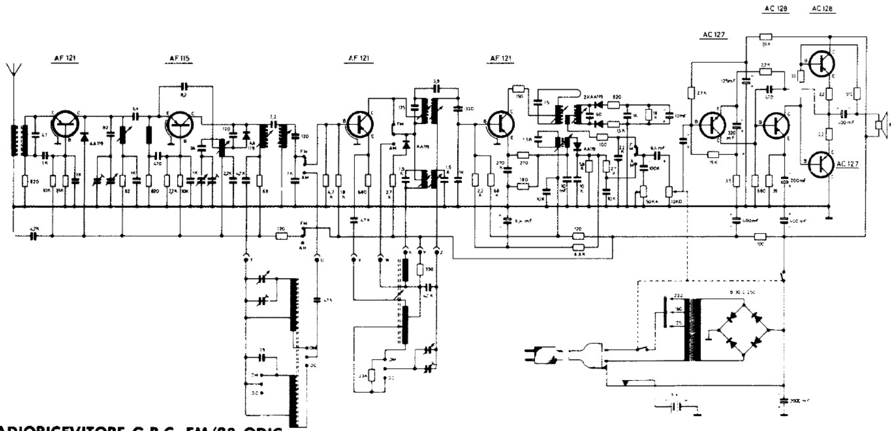
SCHEMA ELETTRICO DEL RADIORICEVITORE G.B.C. FM/38 ODIC
